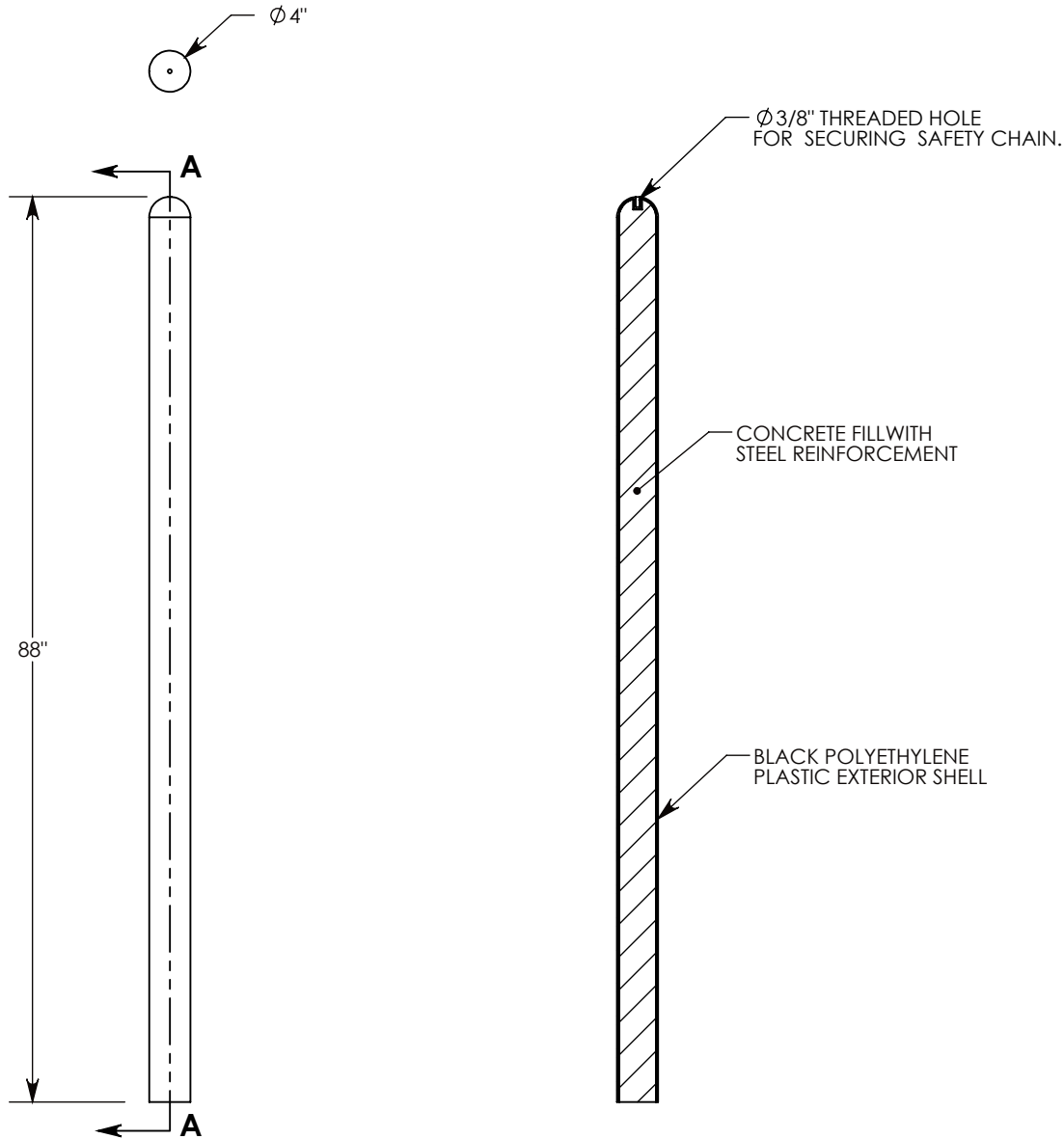
SECTION A-A
