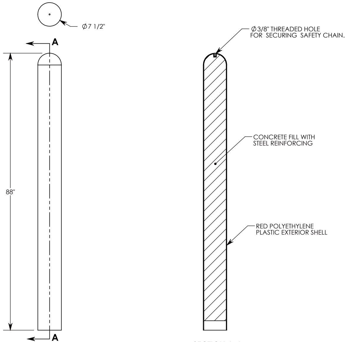
SECTION A-A
