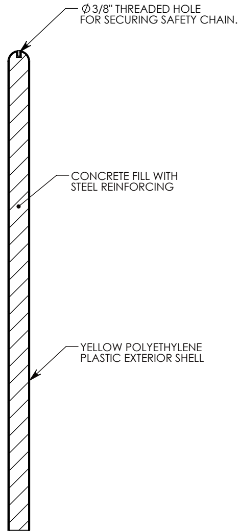
SECTION A-A
