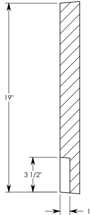
SECTION A-A
