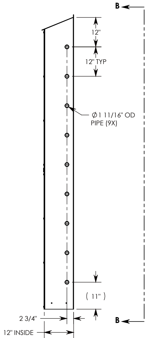
SECTION A-A
