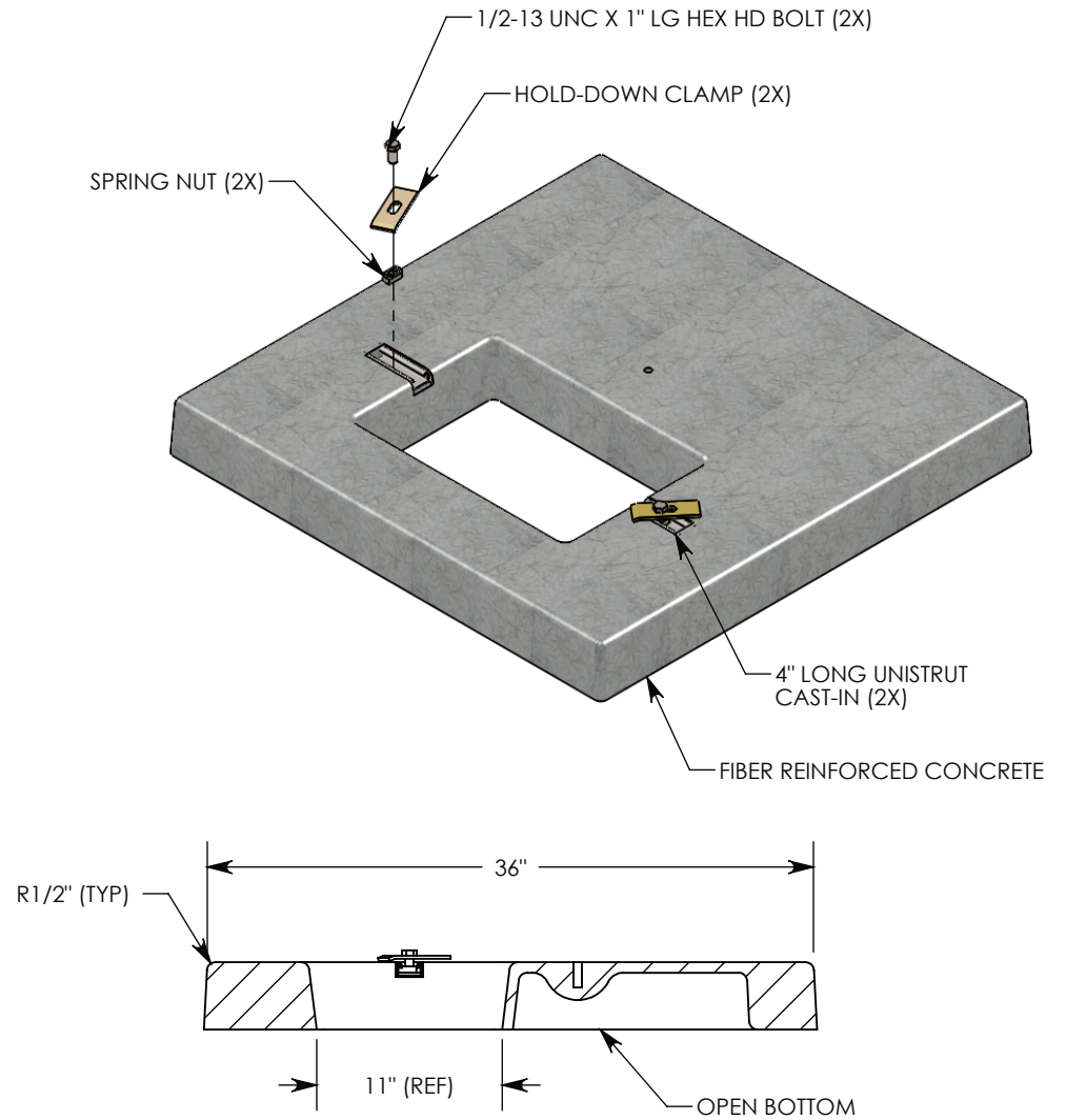
SECTION A-A
