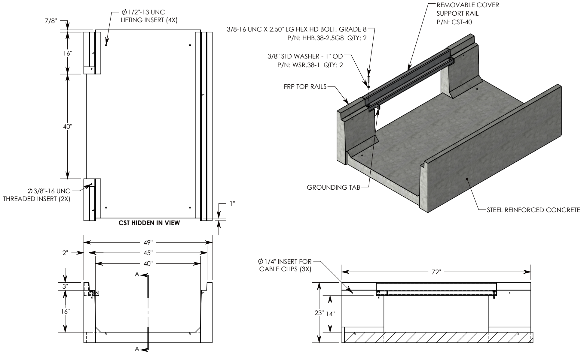
SECTION A-A
