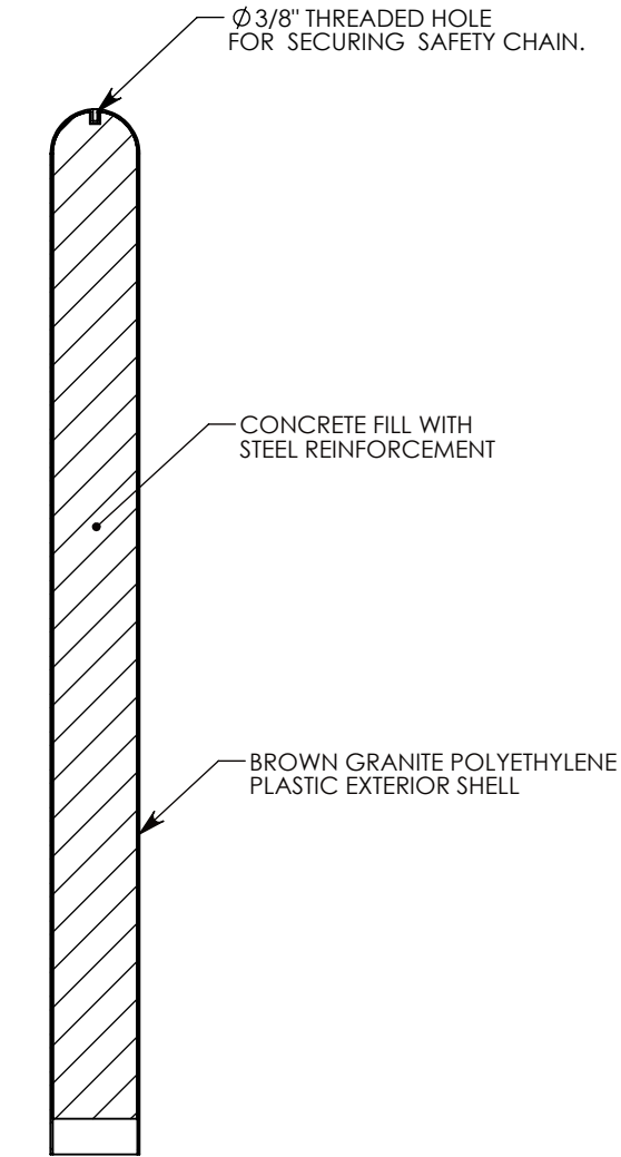
SECTION A-A
