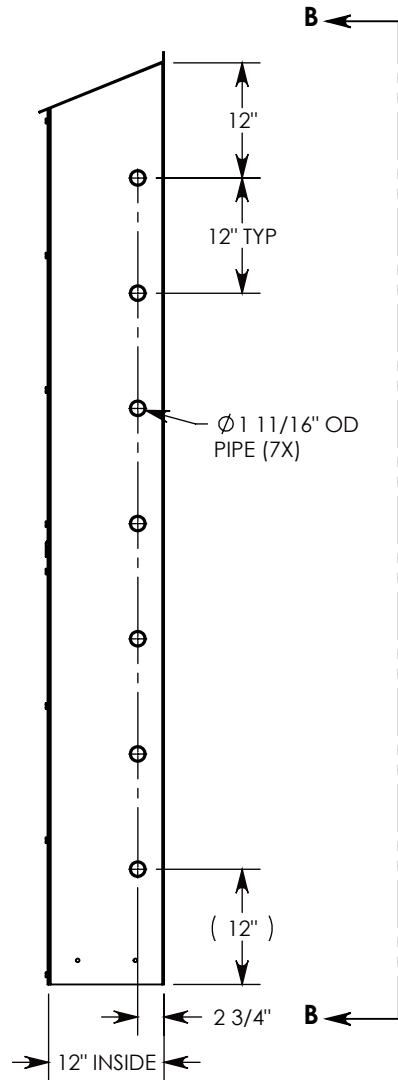
SECTION A-A
